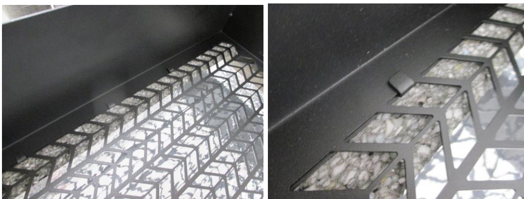
Abbildung 5: Die Blechlasche des Silencers greift in das Gitter des Filterkastens
